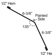
20a GAMBREL FLASHING cccGMBRLH
