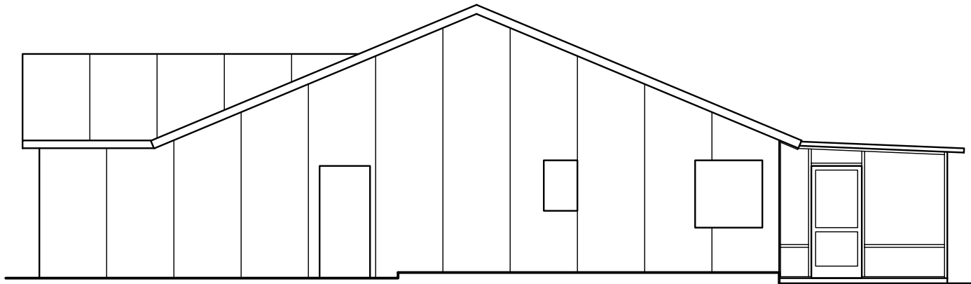
Right Elevation
